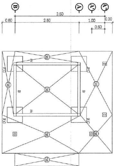
แปลนโครงสร้าง Scale 1:50
