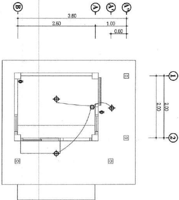
แปลนไฟฟ้า SCALE 1 : 50
